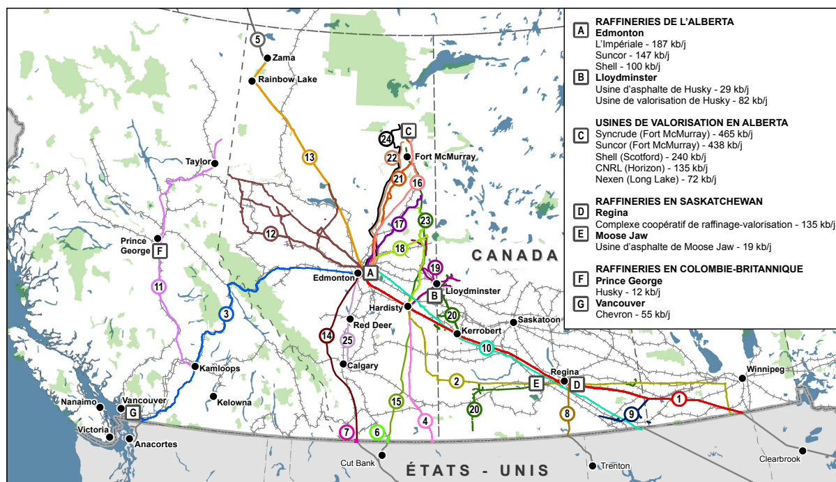
Raffineries et principaux réseaux de transport du pétrole dans l'Ouest canadien
